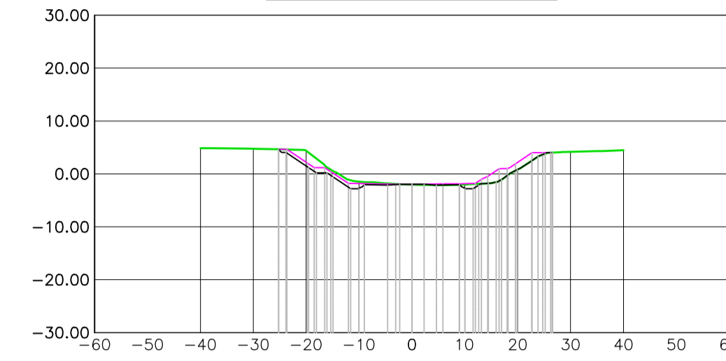
Prog 2575.00 sez 56
