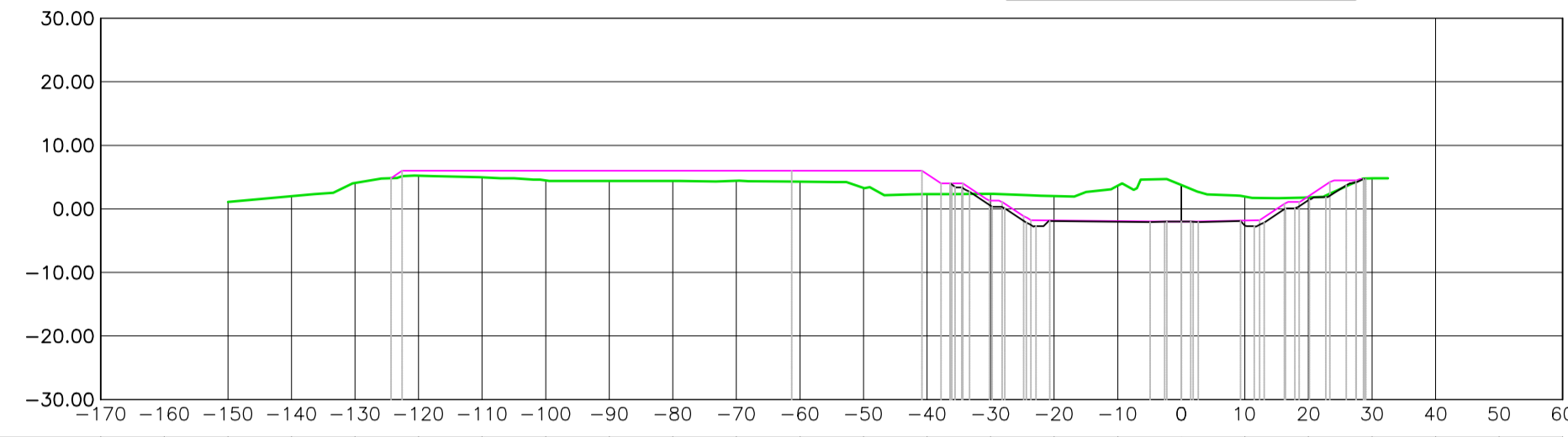
Prog 2050.00 sez 44
