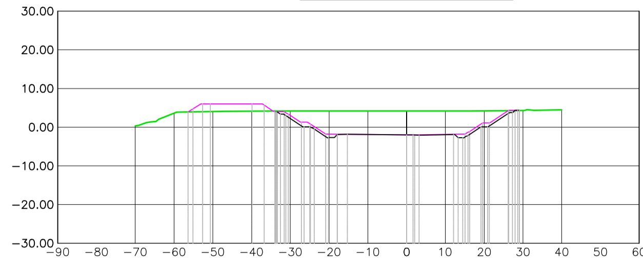
Prog 1850.00 sez 40
