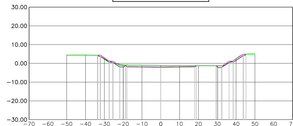
Prog 500.00 sez 11
