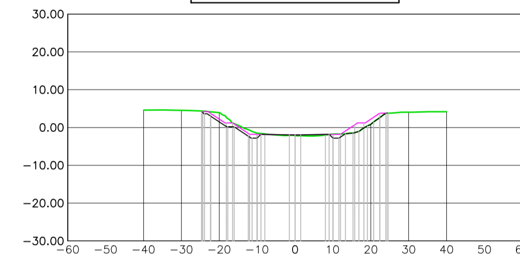
Prog 2700.00 sez 59
