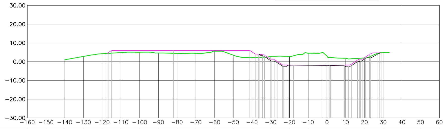
Prog 2100.00 sez 45
