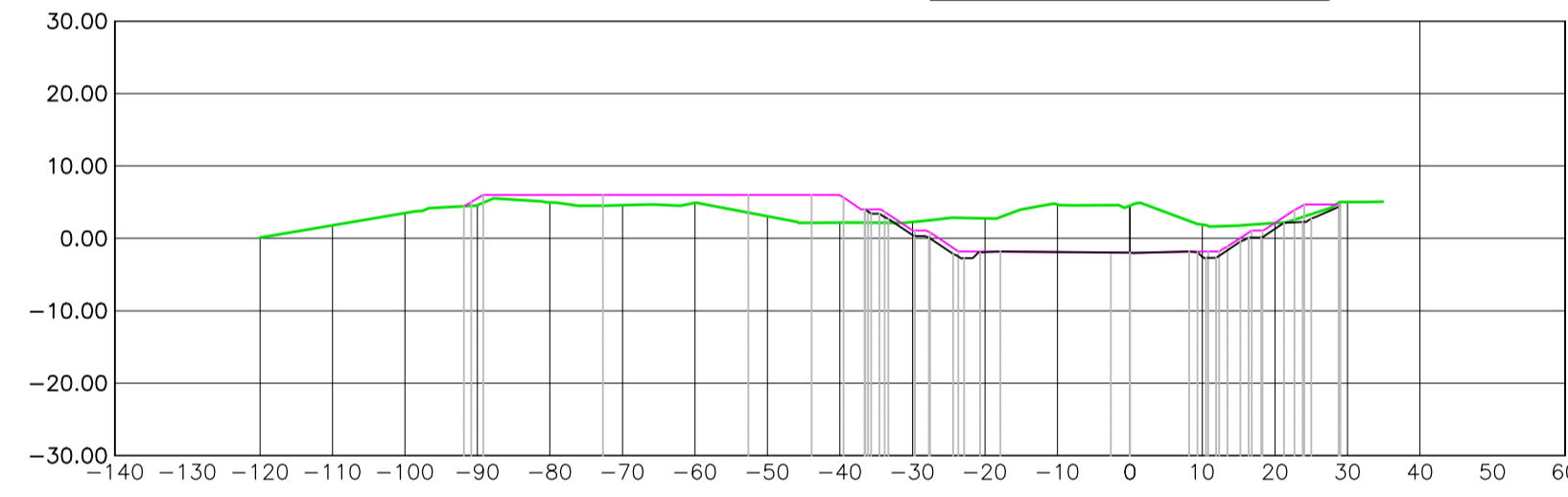
Prog 2150.00 sez 46
