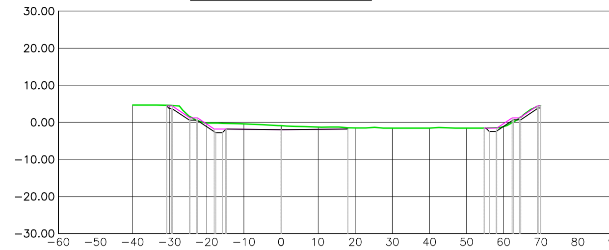
Prog 350.00 sez 8
